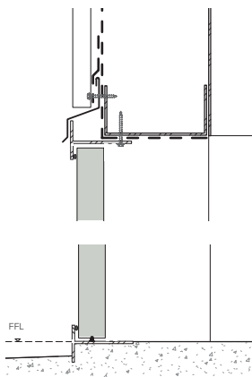
DOOR CROSS SECTION
